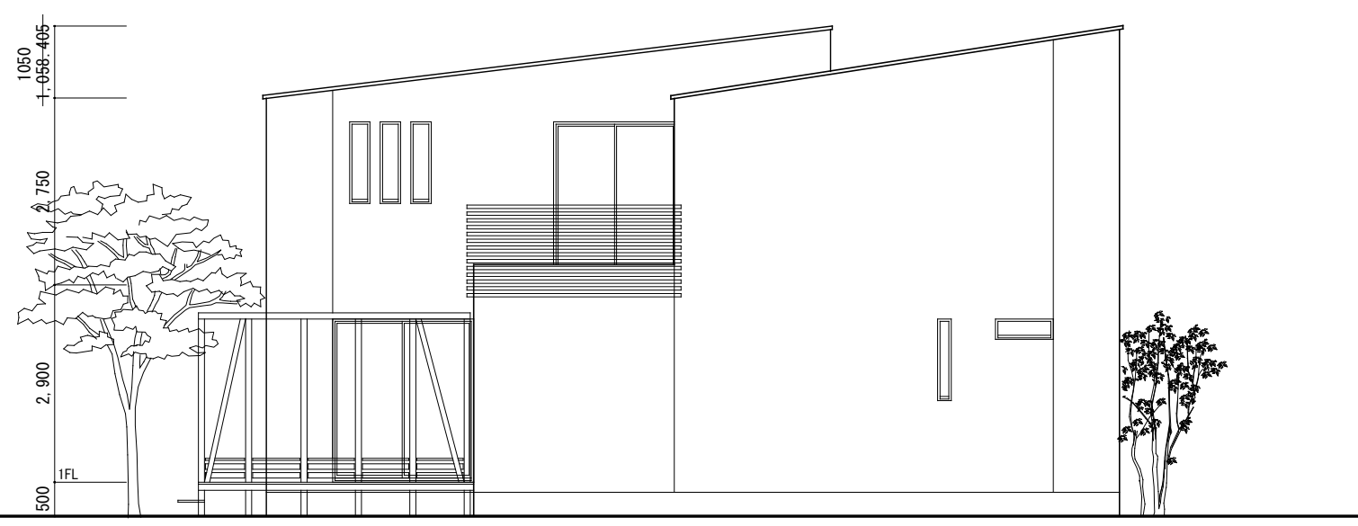
西側 立面
